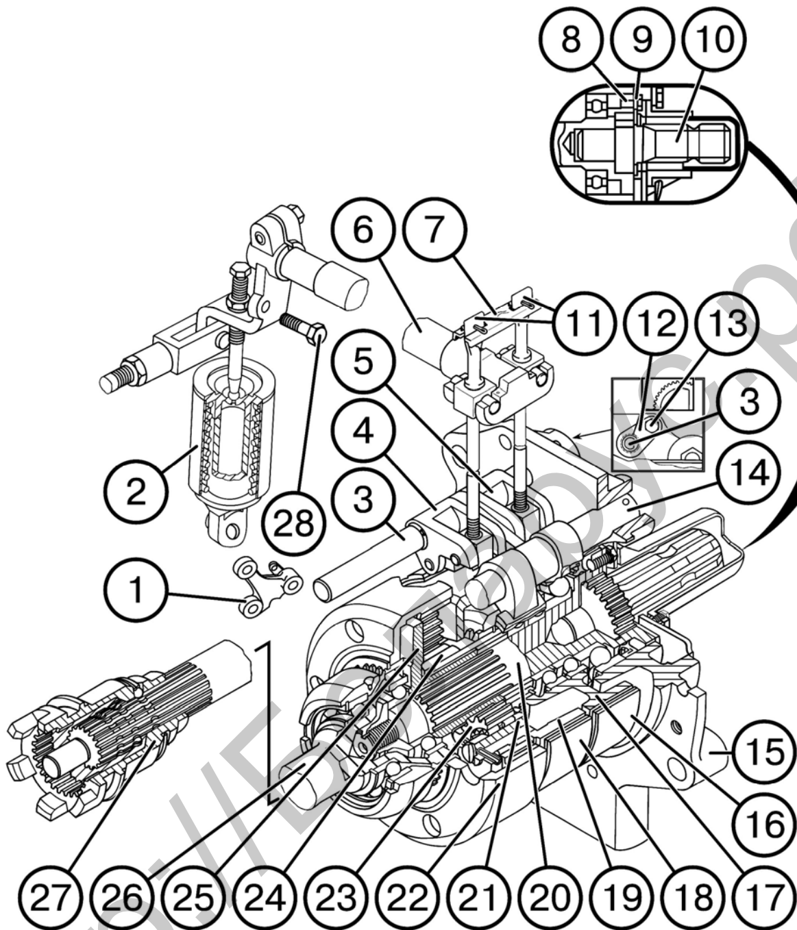
Рис. Д-22. Планетарный редуктор заднего ВОМ:
