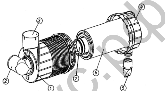
Рис. Д-2. Воздухоочиститель: 1-корпус; 2-патрубок подводящий; 3-воздухозаборник; 4-крышка; 5-резиновый колпак; 6-основной бумажный фильтрующий элемент (ОФЭ); 7-контрольный бумажный фильтрующий элемент (КФЭ).
