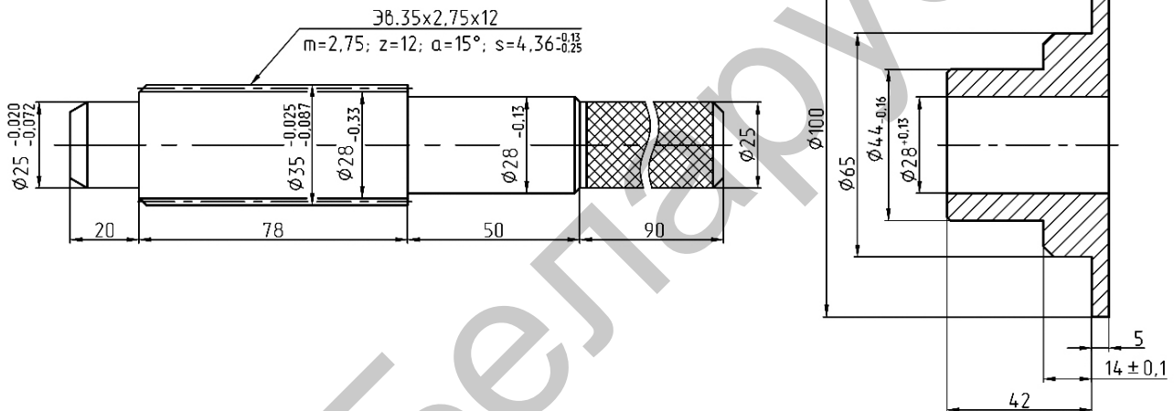
Рис К-10. Технологическая оправка
